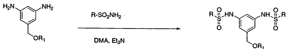
Scheme IV-A
